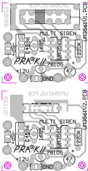
รูปที่4 แสดงลายปริ้นท์และตำแหน่งอุปกรณ์
