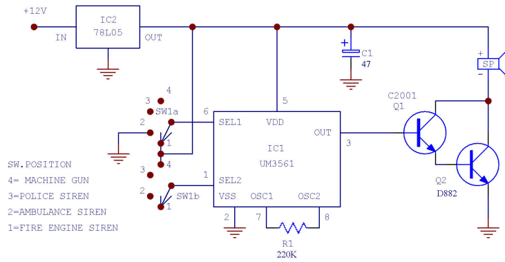
รูปที่3 วงจรมัลติไซเรนที่ใช้งานจริง
