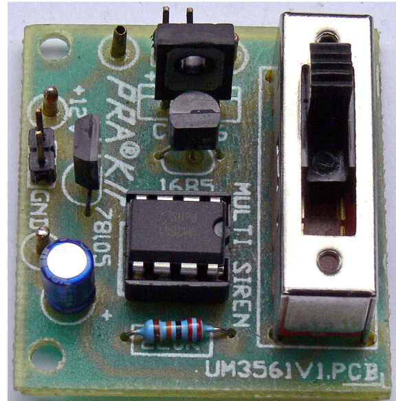
รูปที่ 5 ภาพของจริงเมื่อประกอบเสร็จ
